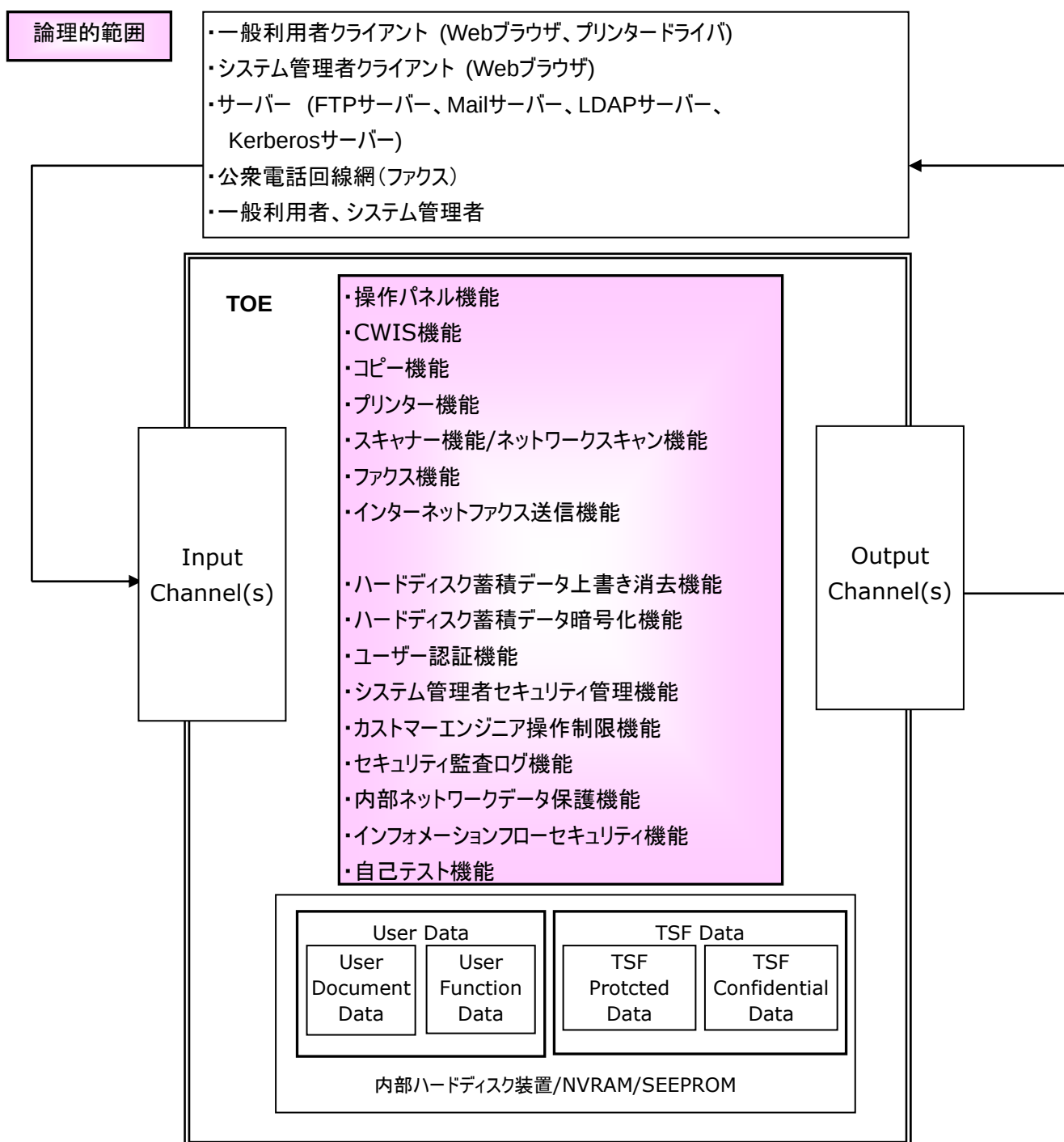
図 2 MFD 内の各ユニットと TOE の論理的範囲
